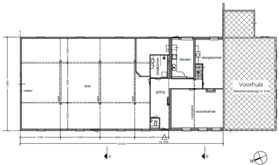
Begane grond
