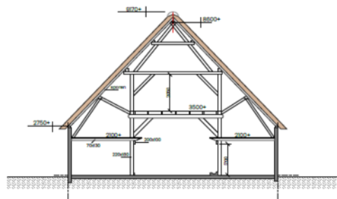
Doorsnede A
