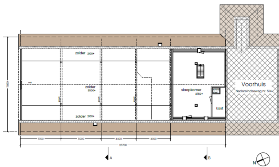
Verdieping
